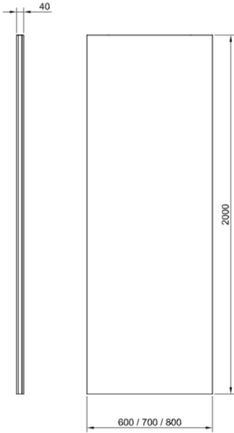
Door dimensions
